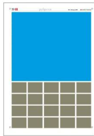
■ 30 модулей (горизонтальный) 250,7 X 218,4 мм
