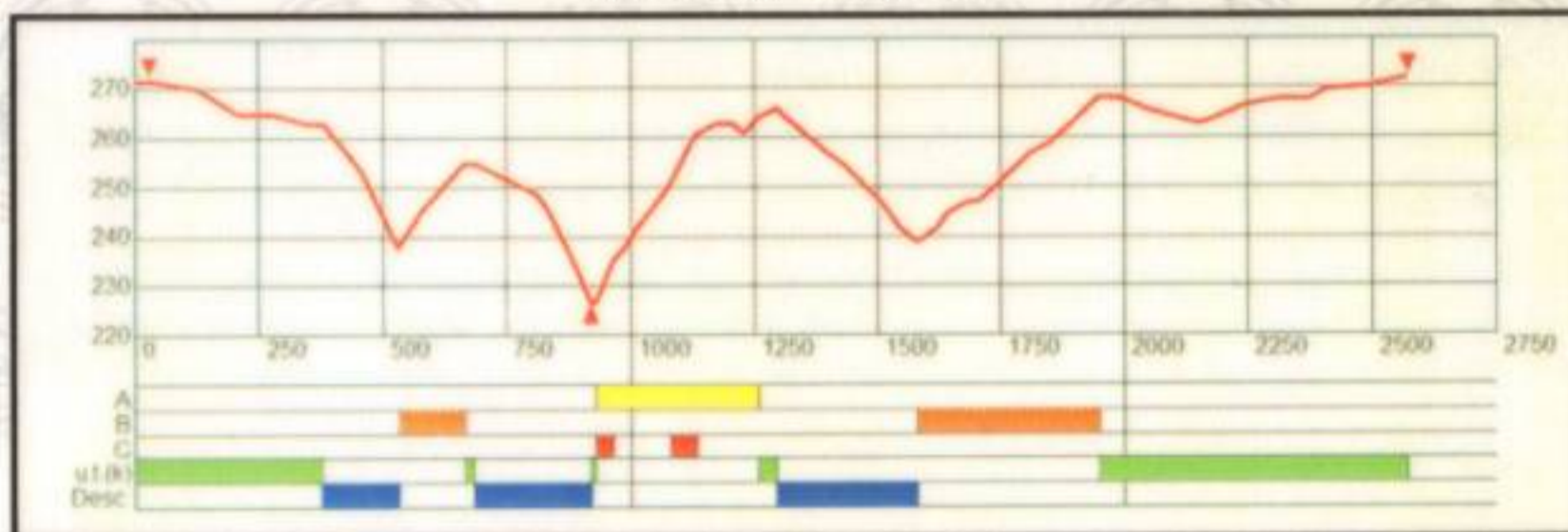
Профиль трассы
