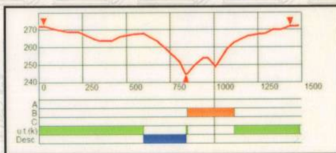
Профиль трассы
