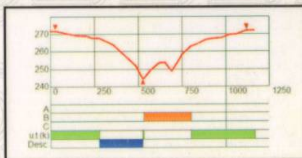
Профиль трассы
